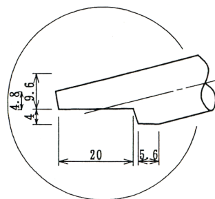
A図（汎用型）
