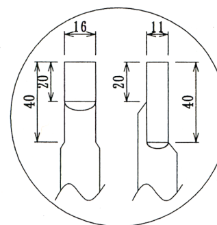
B図（日之出型）
